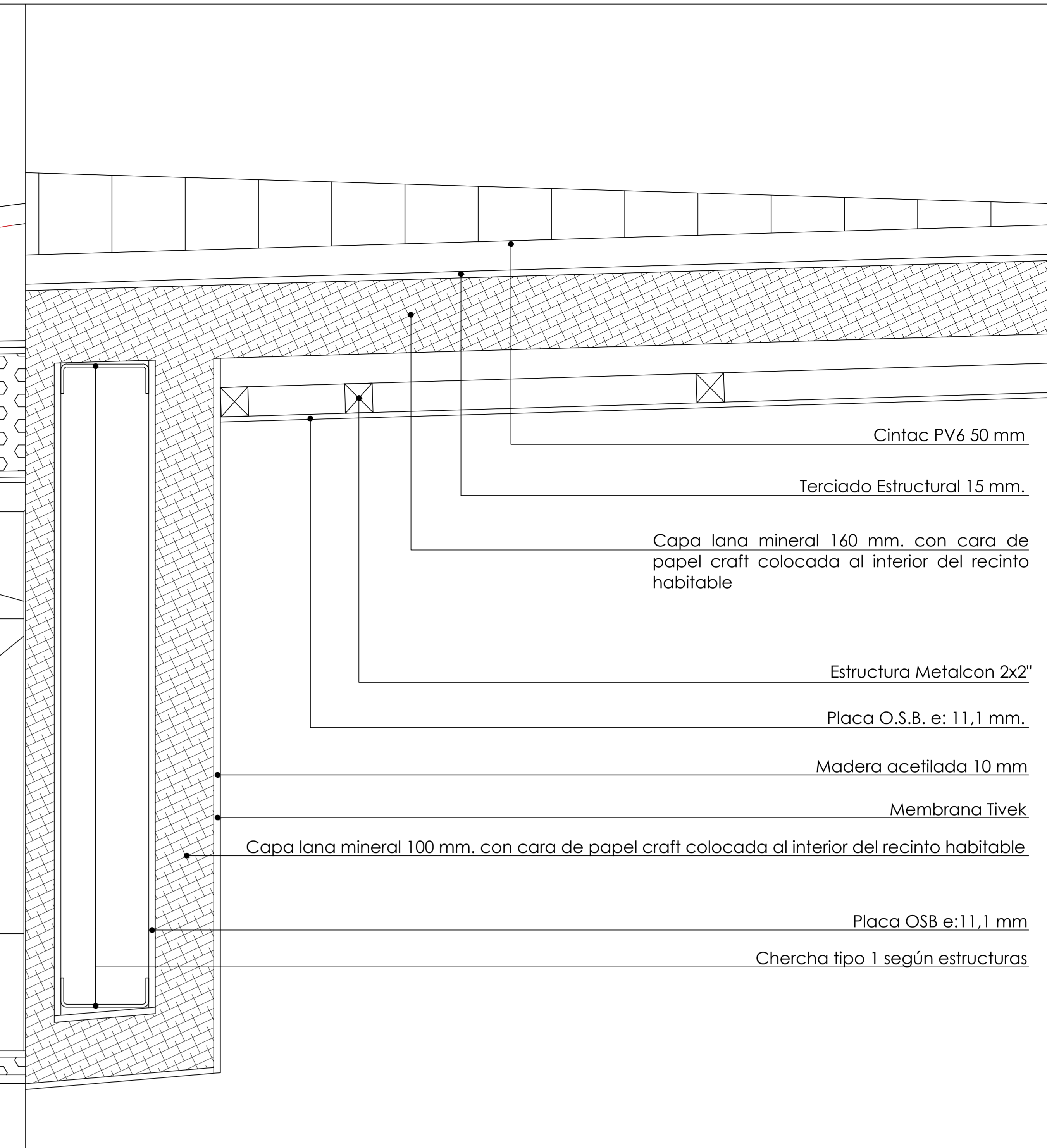
DETALLE CONSTRUCTIVO 3
