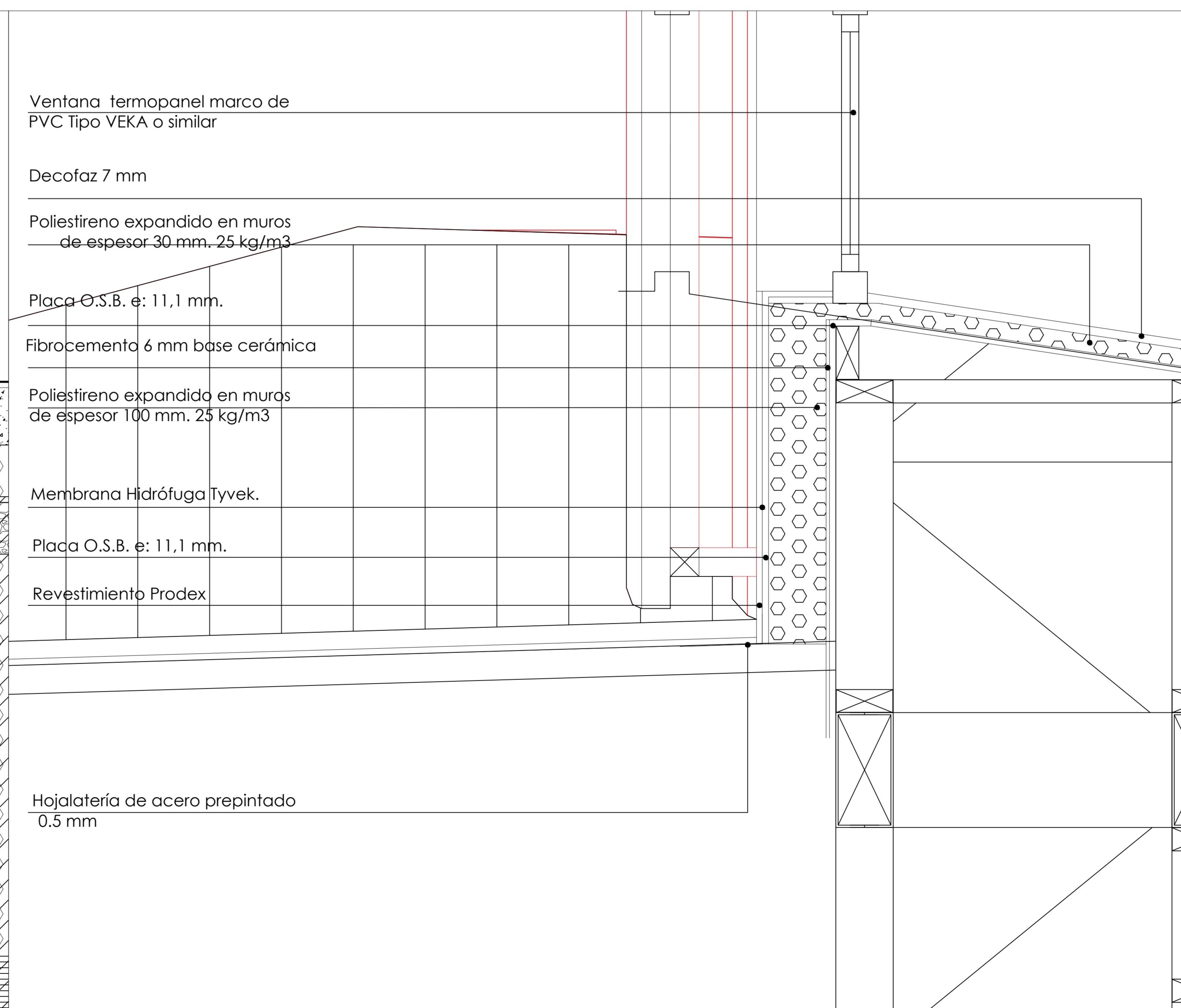
DETALLE CONSTRUCTIVO 5
