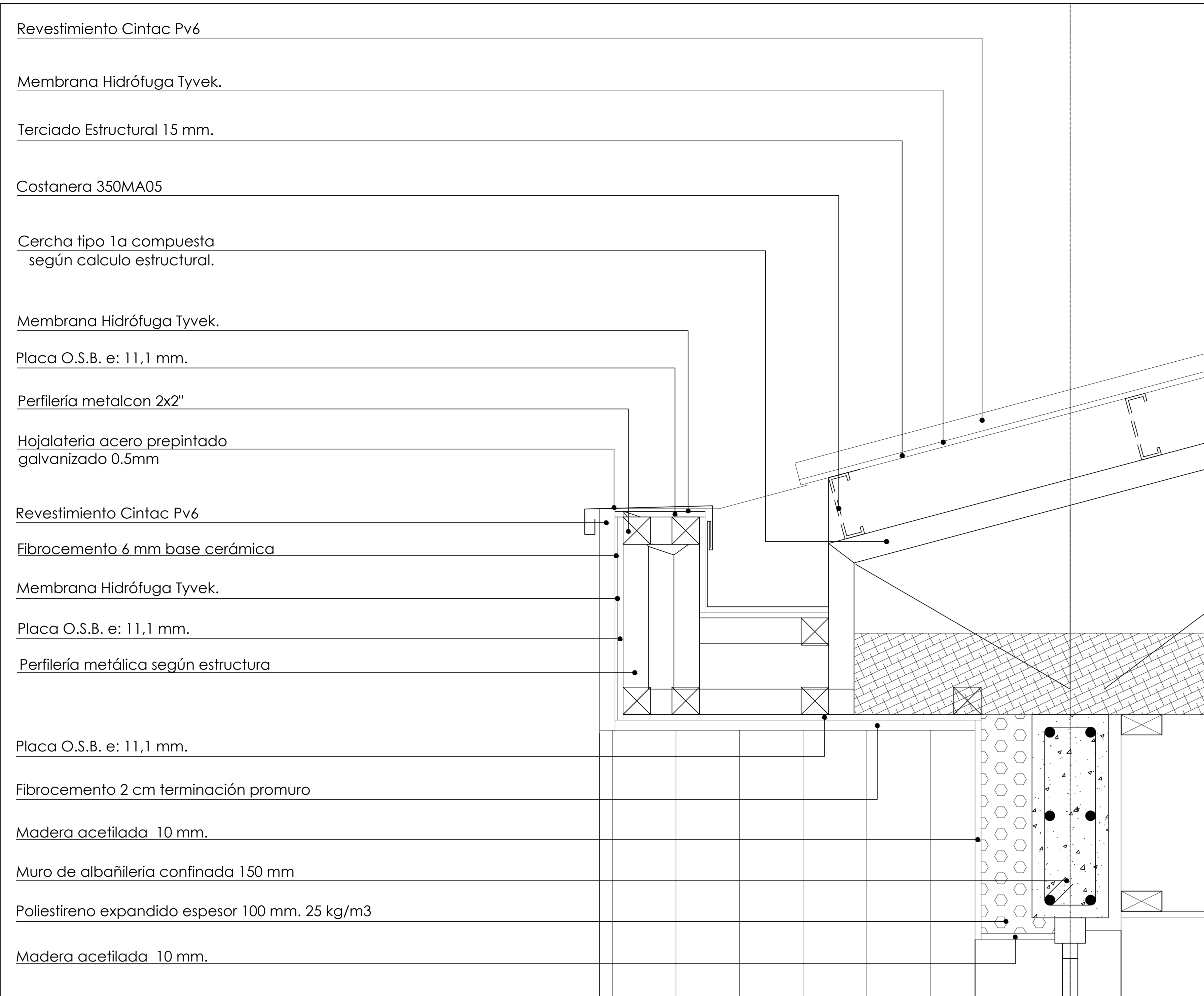
DETALLE CONSTRUCTIVO 1
