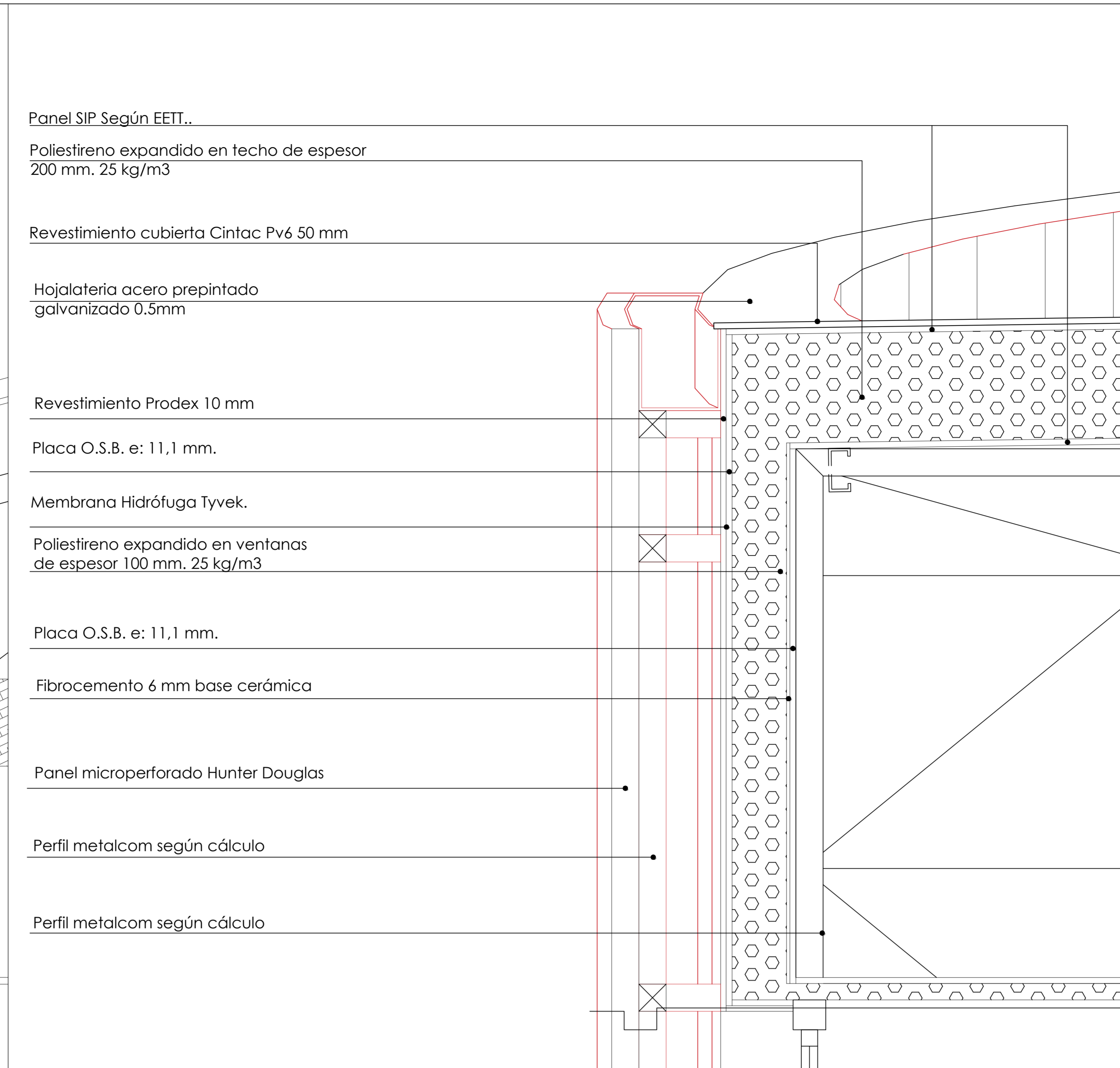
DETALLE CONSTRUCTIVO 2
