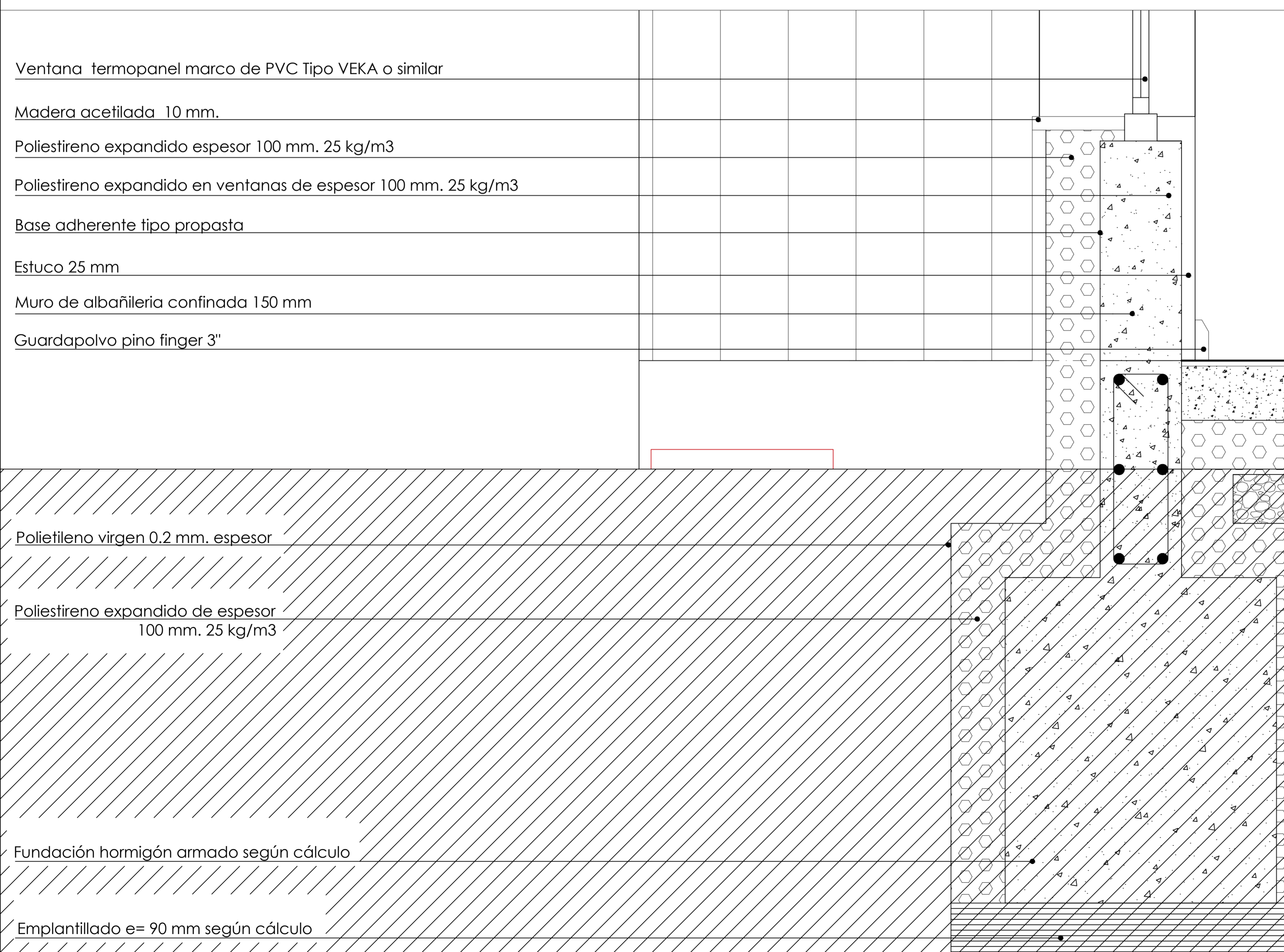
DETALLE CONSTRUCTIVO 4
